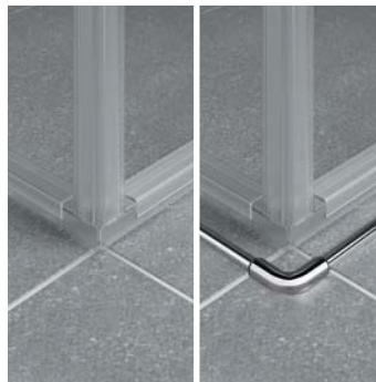
Wahlweise montierbar ohne oder mit kleiner Bodenschwelle zur Verbesserung des Spritzwasserschutzes bei baulichen Gegebenheiten.
