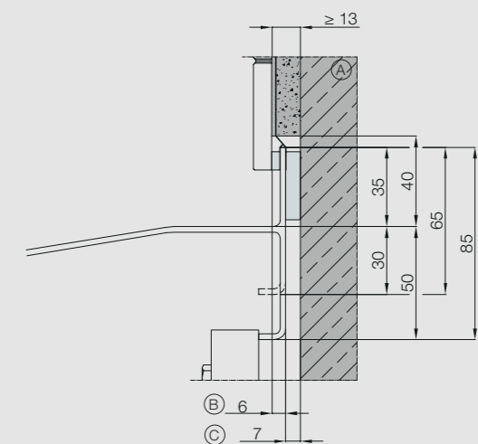
Einbau an der Massivbauwand Installation solid construction
