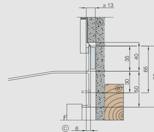
Einbau an der Leichtbauwand Installation lightweight construction
