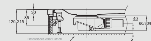
Abb.: mit seitlicher Entwässerung Fig.: with side outlet
