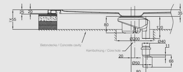
Abb.: mit senkrechter Entwässerung
